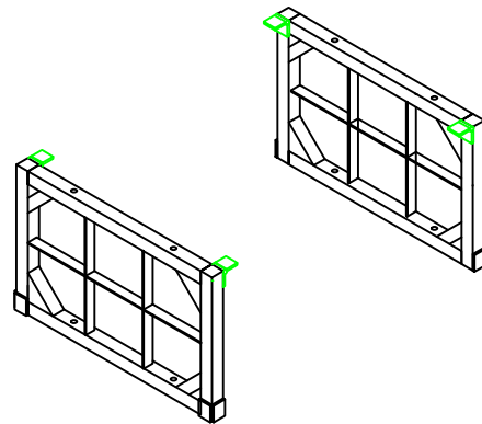
2.2 . Side Frame - 2 Nos.
